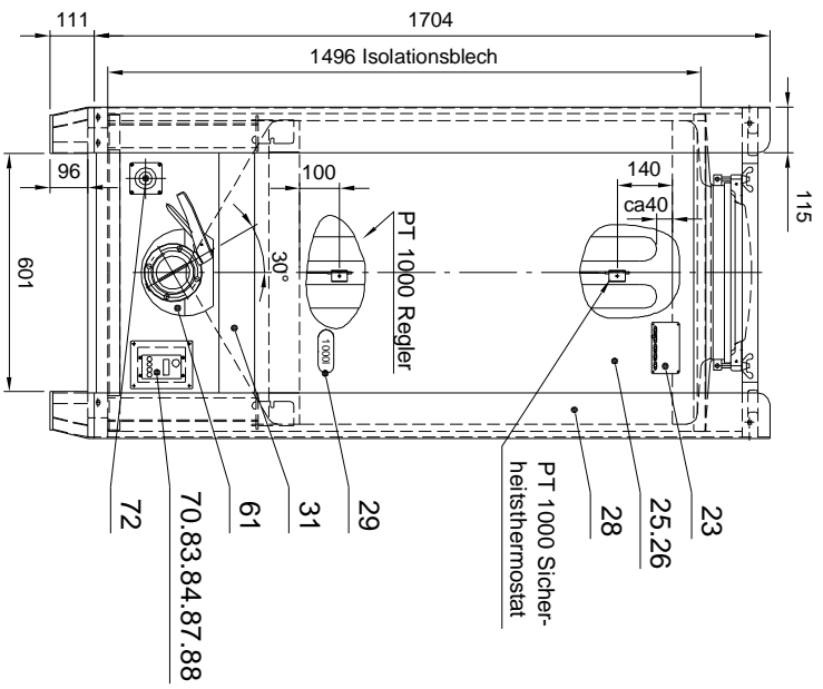
Anordnung PT 1000 + Heizkabel
